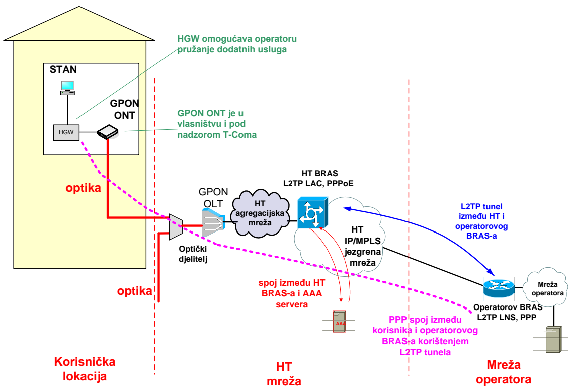
Slika 2. Način realizacije usluge veleprodajnog širokopoasnog pristupa za Internet uslugu na temelju FTTH rješenja na IP razini
