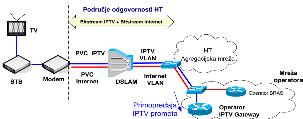
Slika 27. Veleprodajni širokopojsni pristup za pružanje IPTV usluge preko ADSL/VDSL pristupa na DSLAM razini
